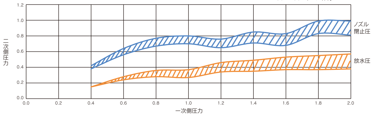
易操作性1号消火栓減圧アダプター付性能曲線(単位:MPa)
